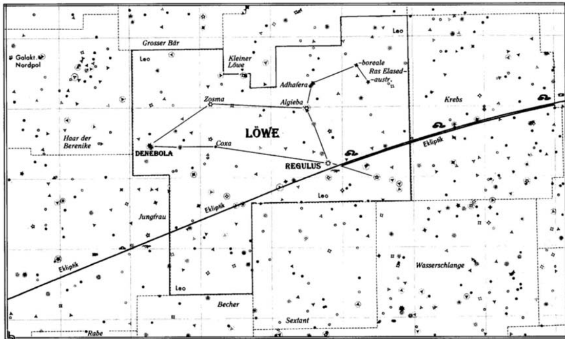
Carta celeste con la constelación de Leo.
